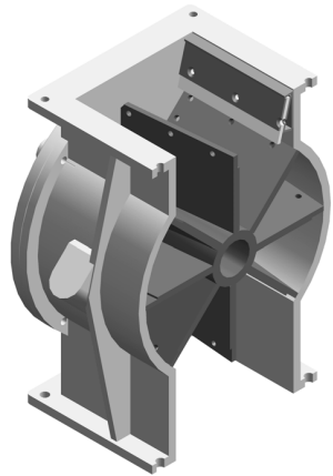
LIMITATORE DI PORTATA SINGOLO / SINGLE SLIP-OFF LIMITEUR DEE PORTÉE / EINLAUFREGULIERUNG
